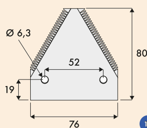
sur-faucillée ép. 3 mm (denture fine)
