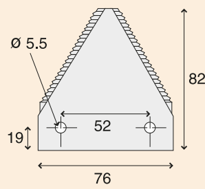
sur-faucillée ép. 2.7 mm
