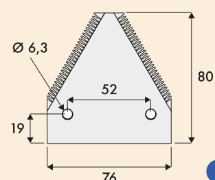
sur-faucillée ép. 3 mm
