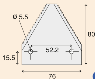
sous-faucillée ép. 2 mm
