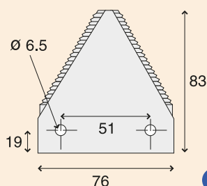
sur-faucillée ép. 2.7 mm
